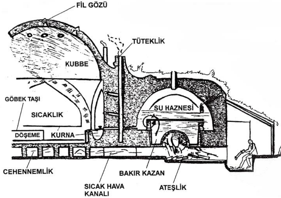
Şekil 11: Külhan Tesisatı.
