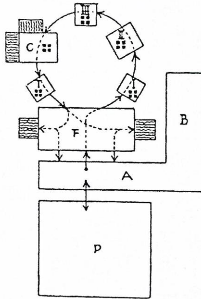
Şekil 8: Asimetrik Hamam Tipi "Pompei Tipi"
