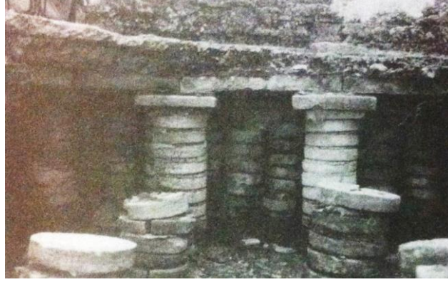
Şekil 6: Yuvarlak sütunla (pilae) hypocaust detayı
