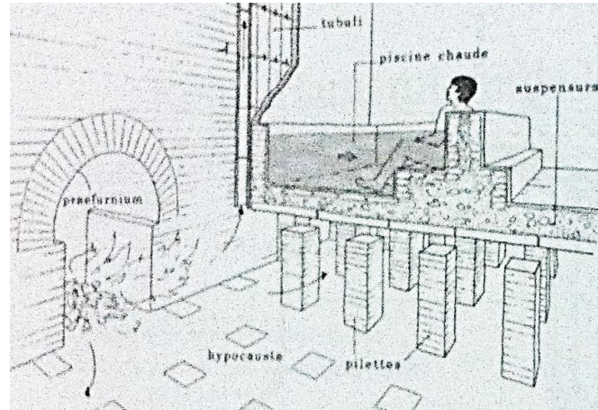
Şekil 5: Pompei Merkez Hamamları ısıtma sistemi
