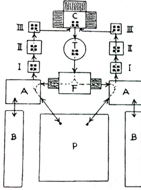
Şekil 7: Simetrik Hamam Tipi "İmparatorluk Hamamları"
