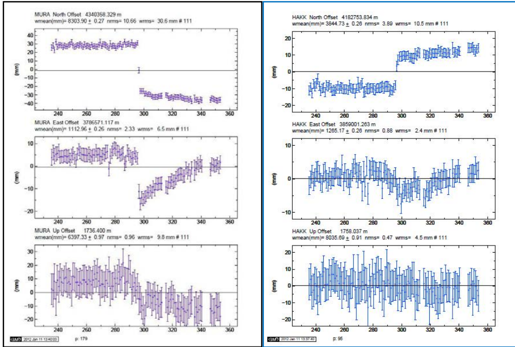
Şekil 5. GNSS veri kullanılarak GAMIT/GLOBK programından MURA ve HAKK istasyonları için elde edilen (a) Kuzey-Güney, (b) Doğu-Batı ve (c) Yükseklik zaman serileri [3].
