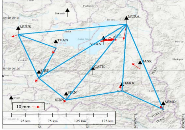
Şekil 6. 7 referans istasyonunun köşe noktası olarak kullanılmasıyla elde edilen 5 üçgen.
