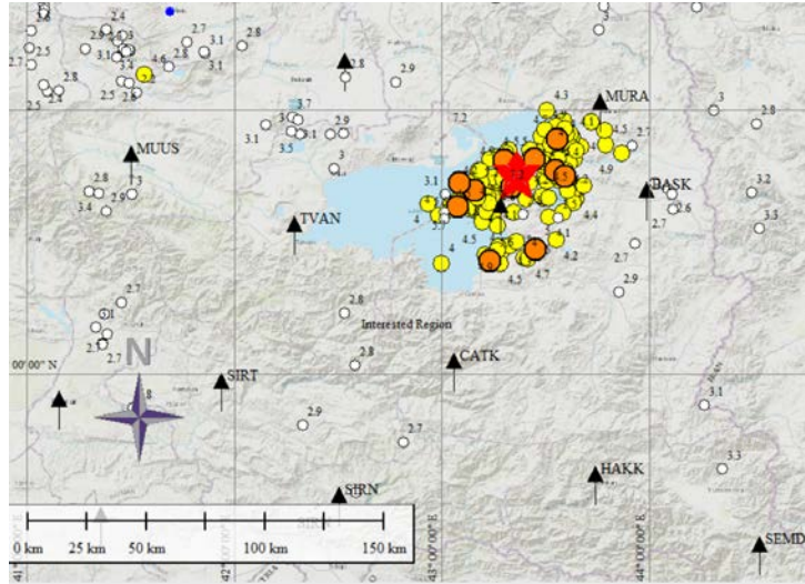
Şekil 2. Deprem bölgesi. Boğaziçi Üniversitesi, Kandilli Rasathanesinden alınan ve deprem gününü de içeren 4 aylık sismik veri şeklinde gösterilmiştir. Burada, beyaz noktalar 2 \leq M \leq 4 , Sarı noktalar 4 \leq M \leq 4.9 , turuncu noktalar 5 \leq M \leq 6 ve Kırmızı yıldız işareti ise 7.2M büyüklüğünde depremleri işaret etmektedir.
